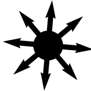
Figura 15 – Estrela do Caos
