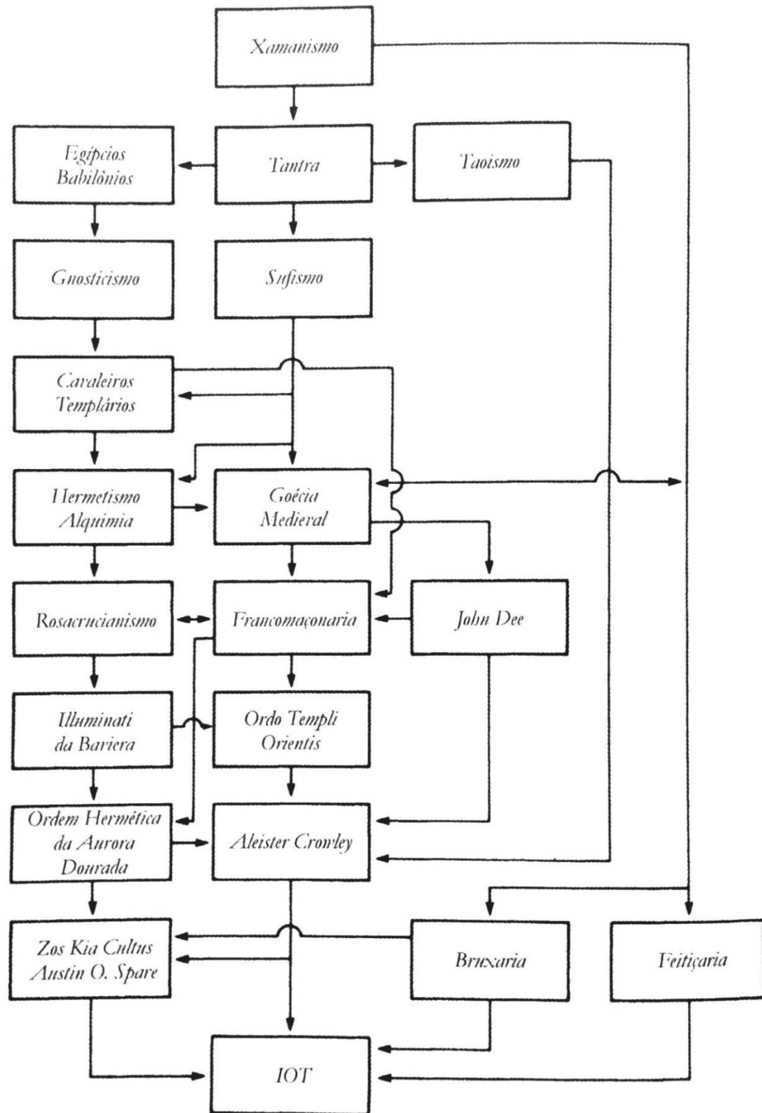
Figura 9 – Diagrama da Sobrevivência da Tradição Mágica
